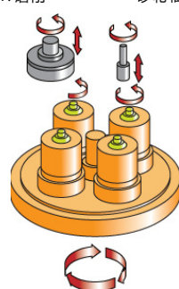
砂轮轴1: 磨削 砂轮轴2: 超精磨
