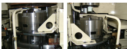
砂轮轴1: 磨削 砂轮轴2: 超精磨
